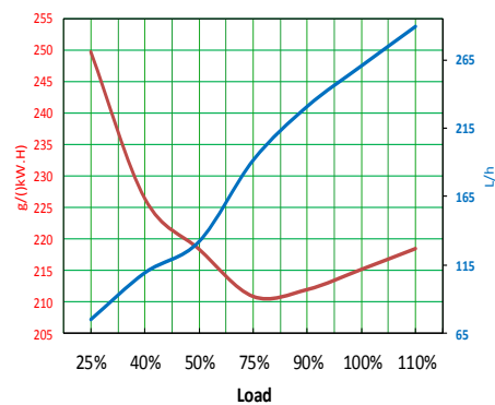
12M26G910/6e2-1014kW/1800rpm
