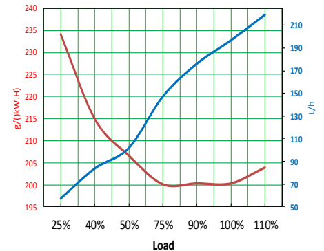
12M26G1000/5e2-820kW/1500rpm
