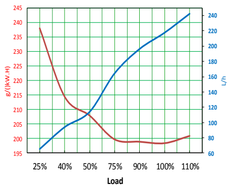
12M26G800/6e2-920kW/1800rpm
